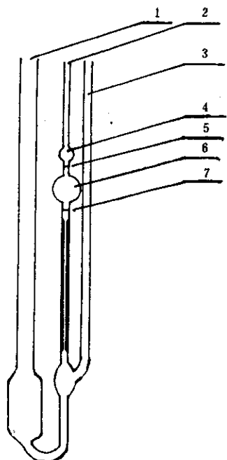
图 2 非稀释型乌氏粘度计
