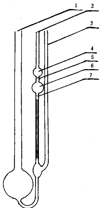
图 1 稀释型乌氏粘度计
